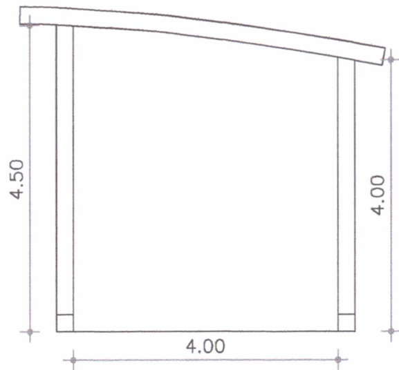
02 CORTE AA ESCALA = 1:75
