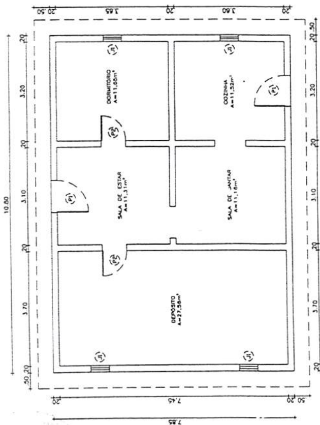
① PLANTA BAIXA SEM ESCALA
