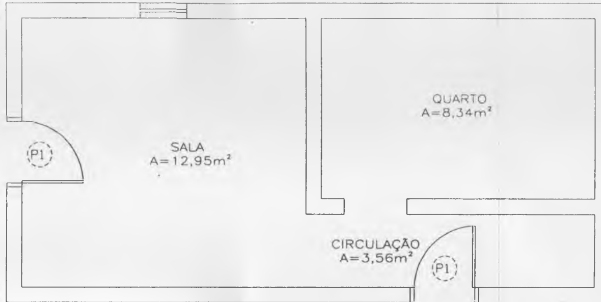
1 PLANTA BAIXA ESC 1/50
