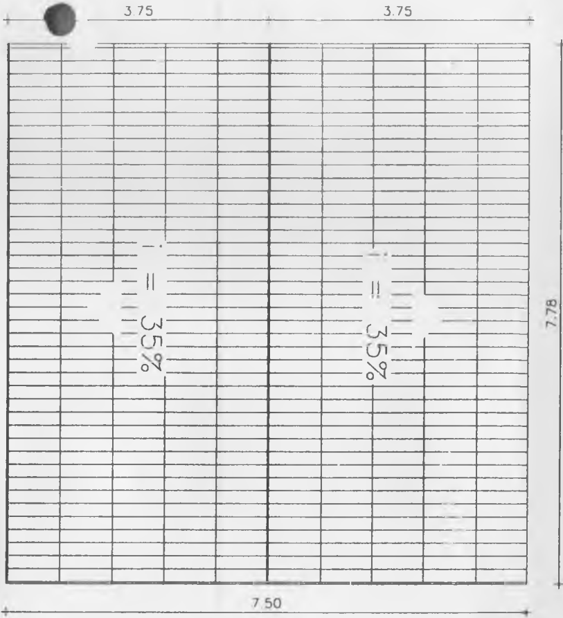
② PLANTA DE COBERTA ESC 1/75
