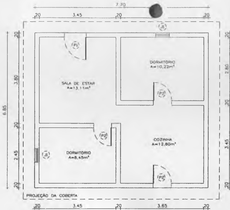
1 PLANTA BAIXA SEM ESCALA
