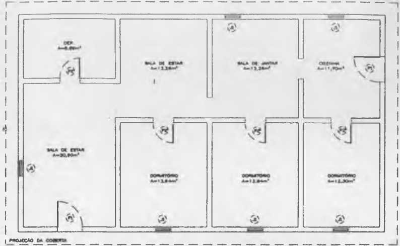
1 PLANTA BAIXA SEM ESCALA
