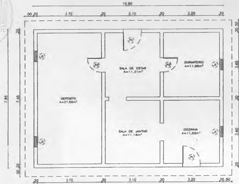
1 PLANTA BAIXA SEM ESCALA
