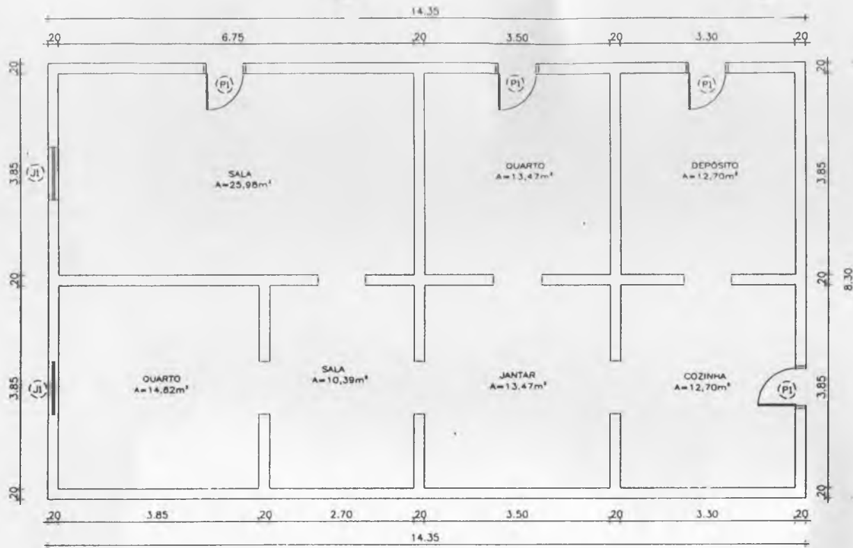
1 PLANTA BAIXA ESC 1/100
