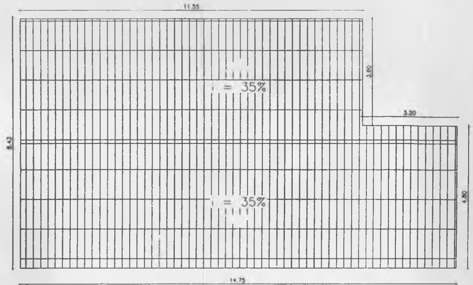
2 PLANTA DE COBERTA SEM ESCALA
